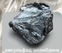
дисульфид молибдена
